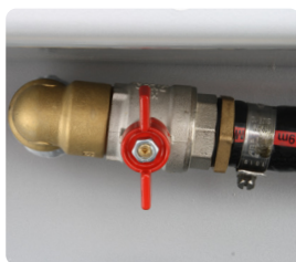
Montiertes Kugelventil und Schlauchnippel 3/4" Anschluss.
